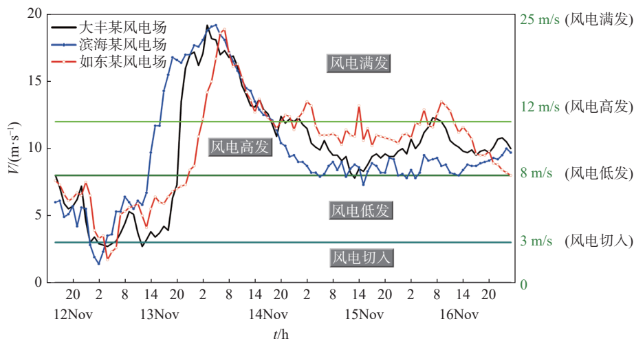
图 4 江苏海上风电发电气象条件预报曲线(2023 年 11 月 12 日 16 时—16 日 04 时)
