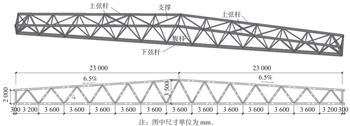
图 3 单榀横向桁架视图 Fig. 3 View of single transverse truss
