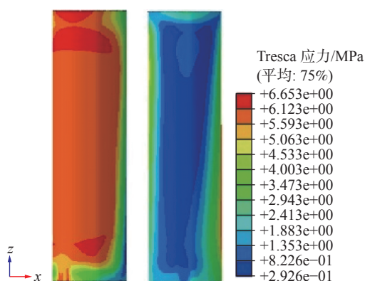
图 6 灌浆体 Tresca 应力
