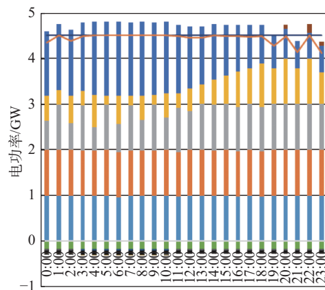
注: 火电 #1 出力; 火电 #4 出力; 火电 #3 出力; 火电 #4 出力; 风电出力; 厂用电负荷; 储能充电; 储能放电; 制氢耗电; 制氢耗电; 通道容量; 送出需求。
