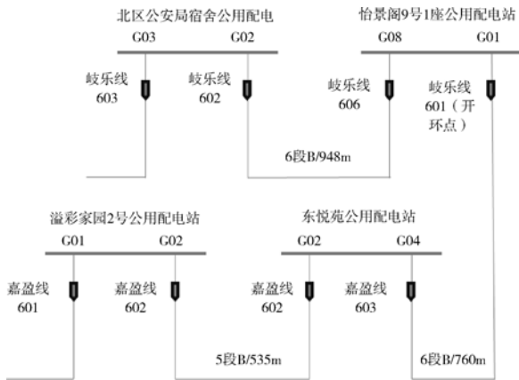
图 2 线路运行方式图
