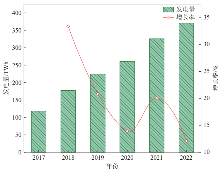
图8 2017—2022年中国光伏发电量情况 [32]
