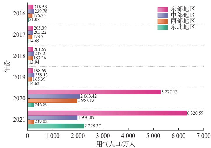
图 2 2016—2021 年中国农村燃气使用人口分布情况 [12]
