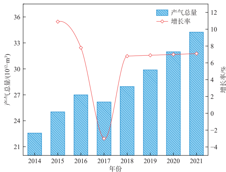
图 5 2014—2021 年中国农村沼气工程产气总量 [25]
