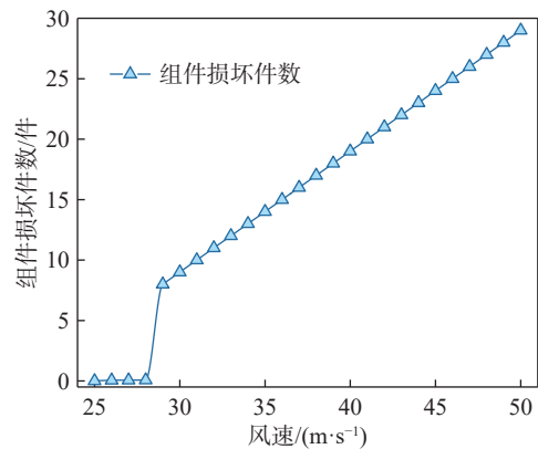
图 6 不同风速下光伏组件破损分析
