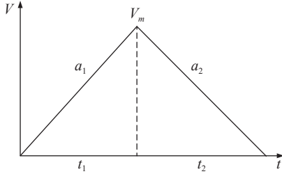
图 3 三角形速度曲线
