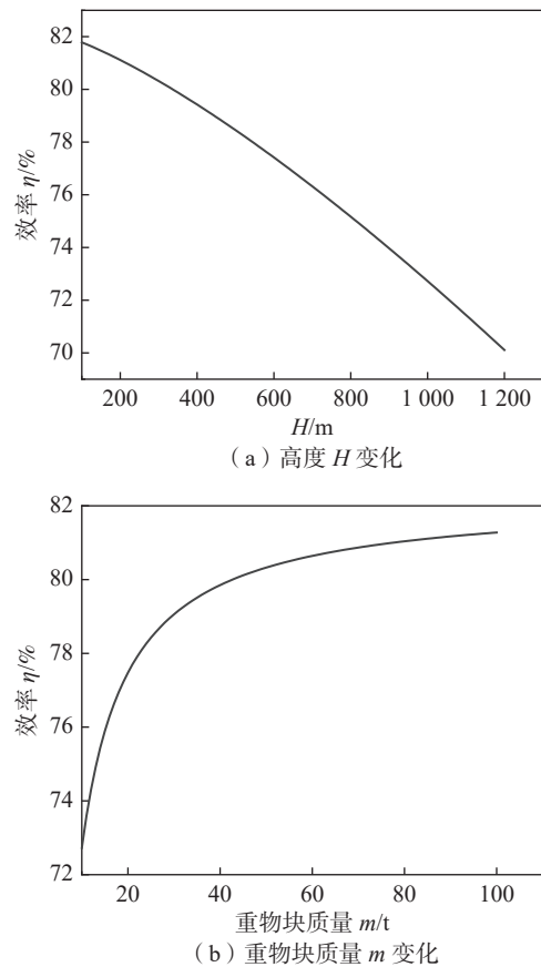
图10 不同高度、重物块质量下的发电效率变化
