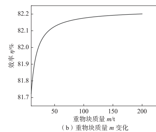
图 8 不同高度、重物块质量下的发电效率变化
