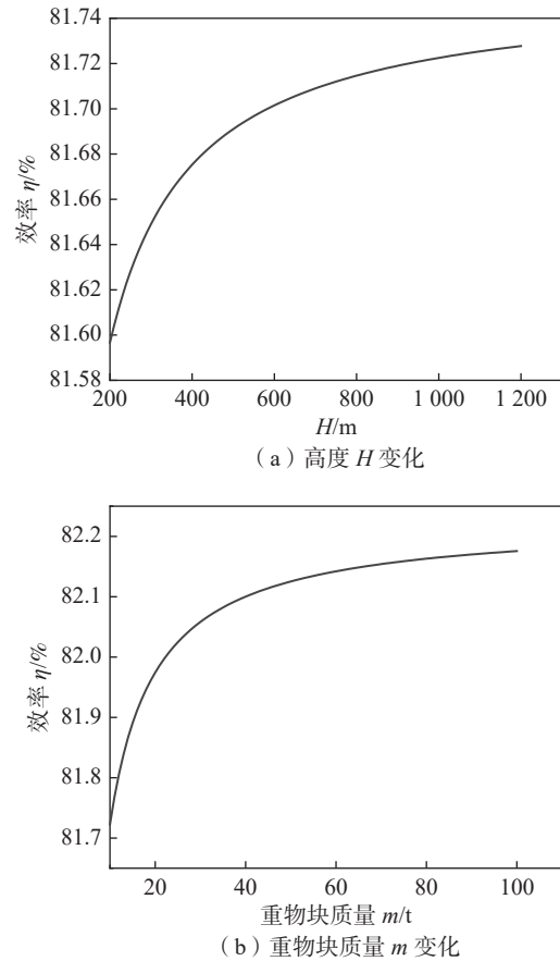
图6 不同高度、重物块质量下的发电效率变化
