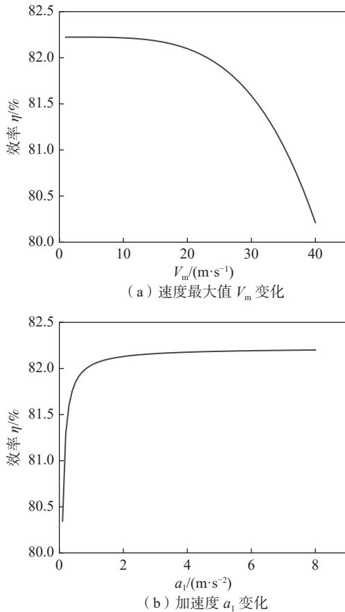
图5 不同速度下的发电效率变化
