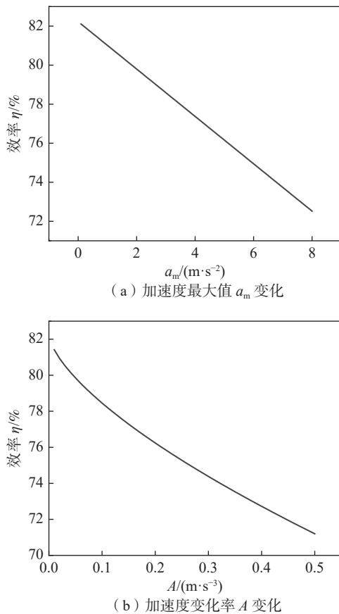
图9 不同速度下的发电效率变化
